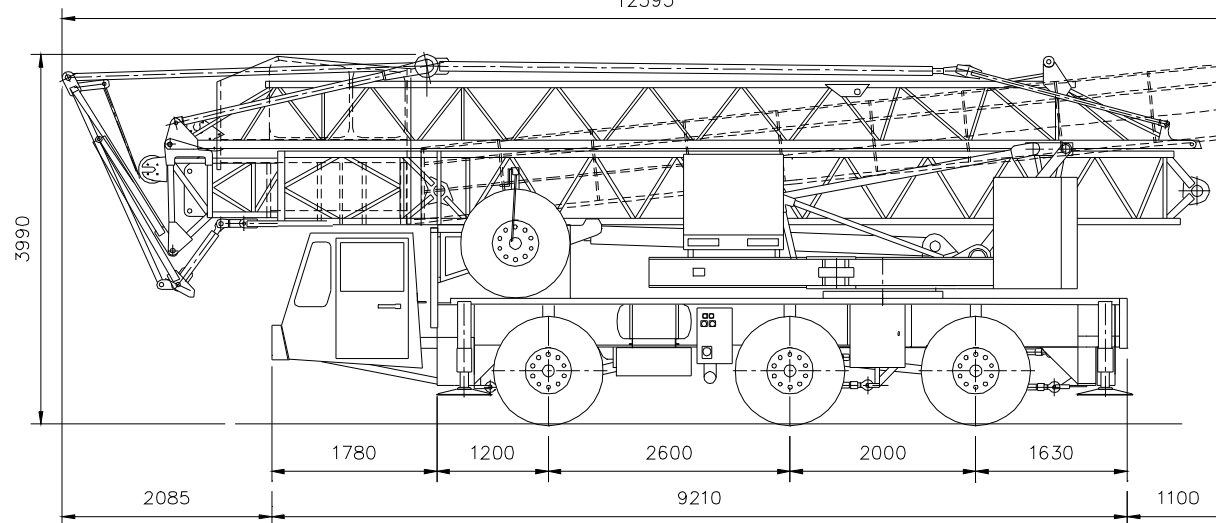
SPIERINGS VOUWKRAAN SK345-AT3
